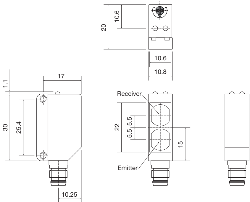
Fig. 6 Plug
